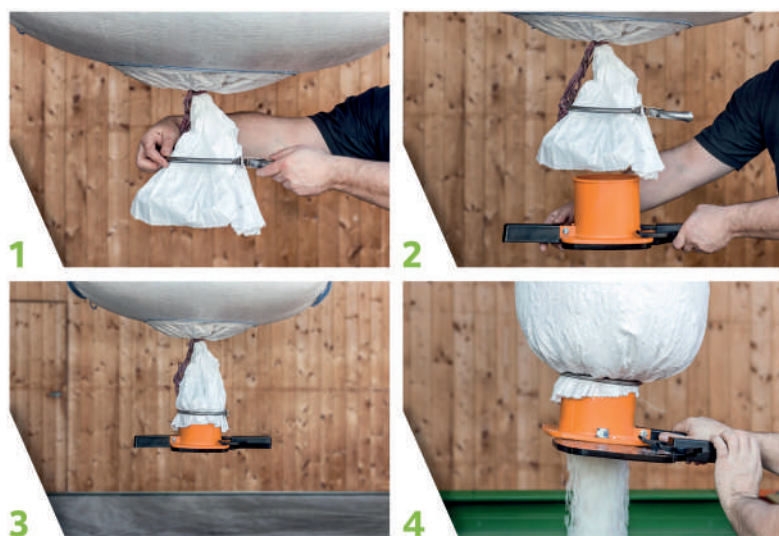
Montaje StackPack Dosificador Easy
