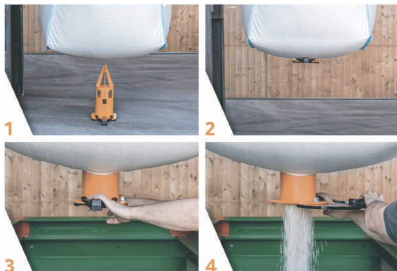
Montaje StackPack Dosificador Original
